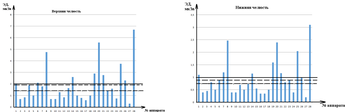
Рис. 3. Гистограмма распределения эффективных доз при рентгенографии резцов верхней челюсти; — — стандартизированная средняя доза, - - - -75 % квантиль, - · - · -50 % квантиль
